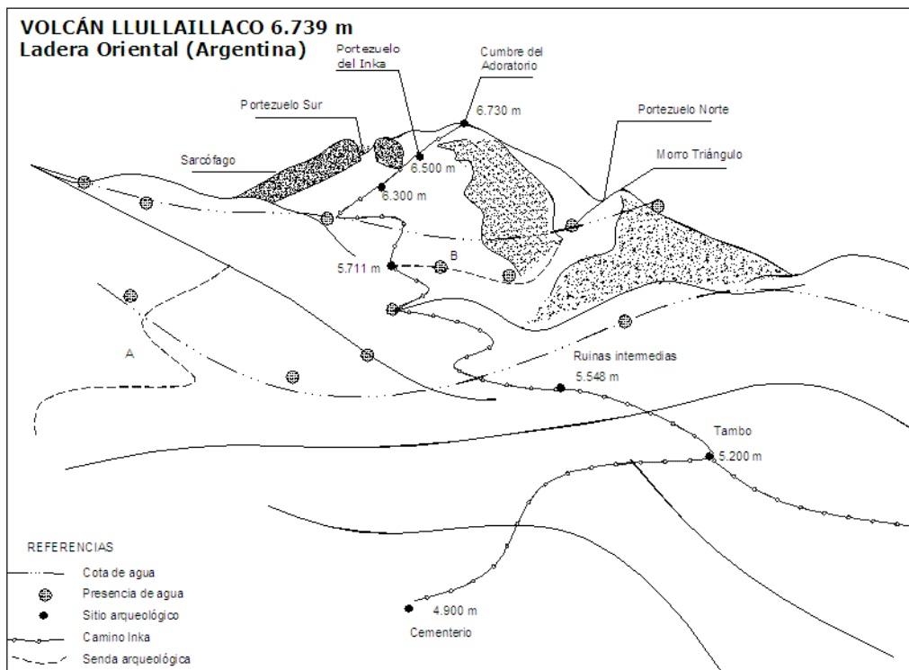
Dibujo 1: Volcán Lullailaco visto desde su vertiente NE. Se aprecian las principales geformas que lo definen, las sendas relacionadas con los sectores de obtención de agua (A y B), los caminos y sitios asociados ubicados en diferentes cotas altitudinales.
